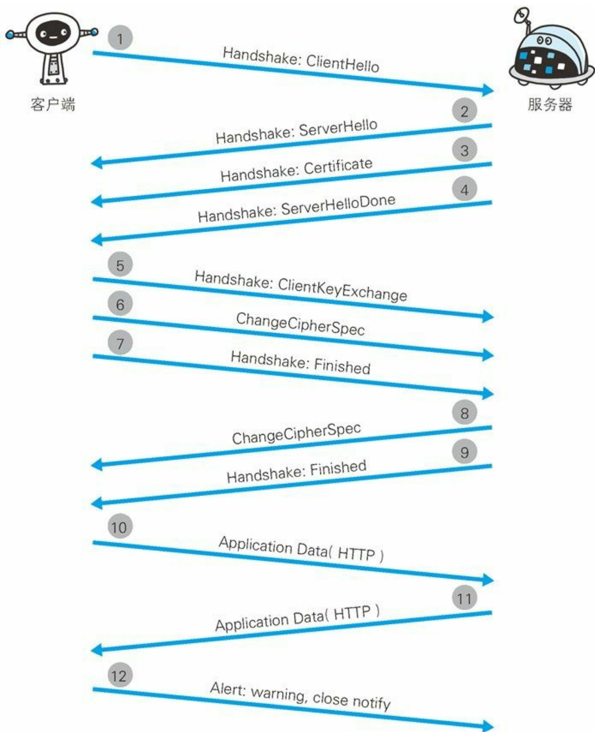
图：HTTPS 通信
