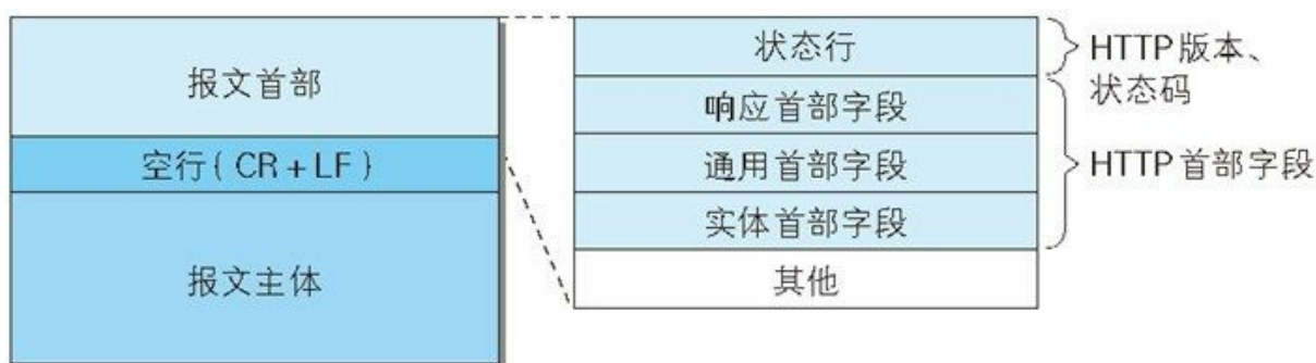
图：响应报文
